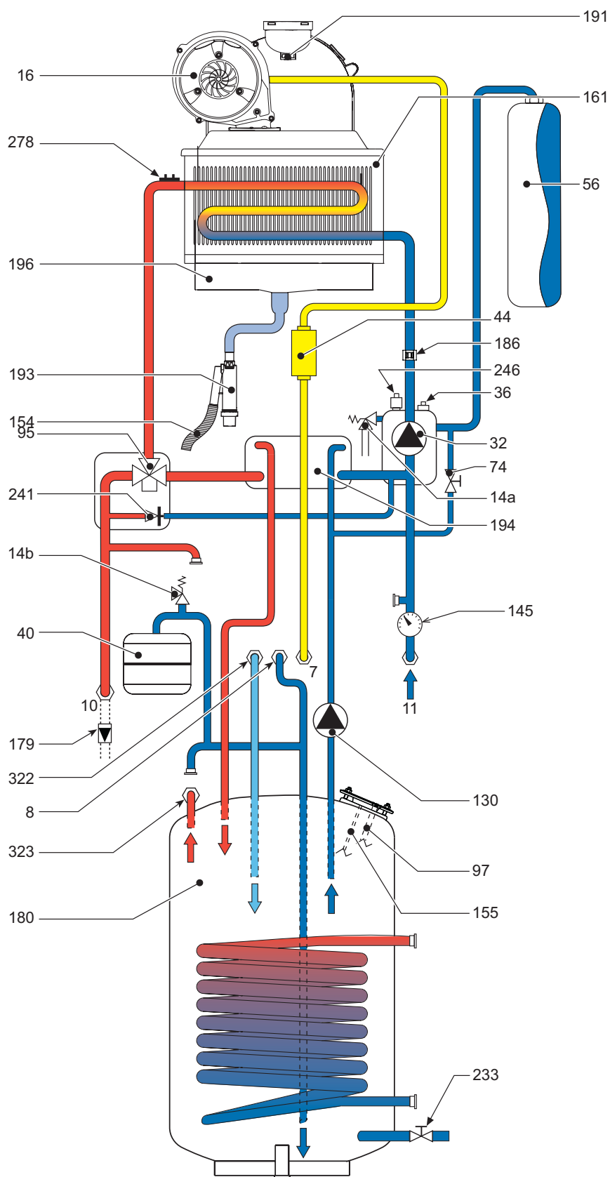
fig. 45 - Circuito idraulico
