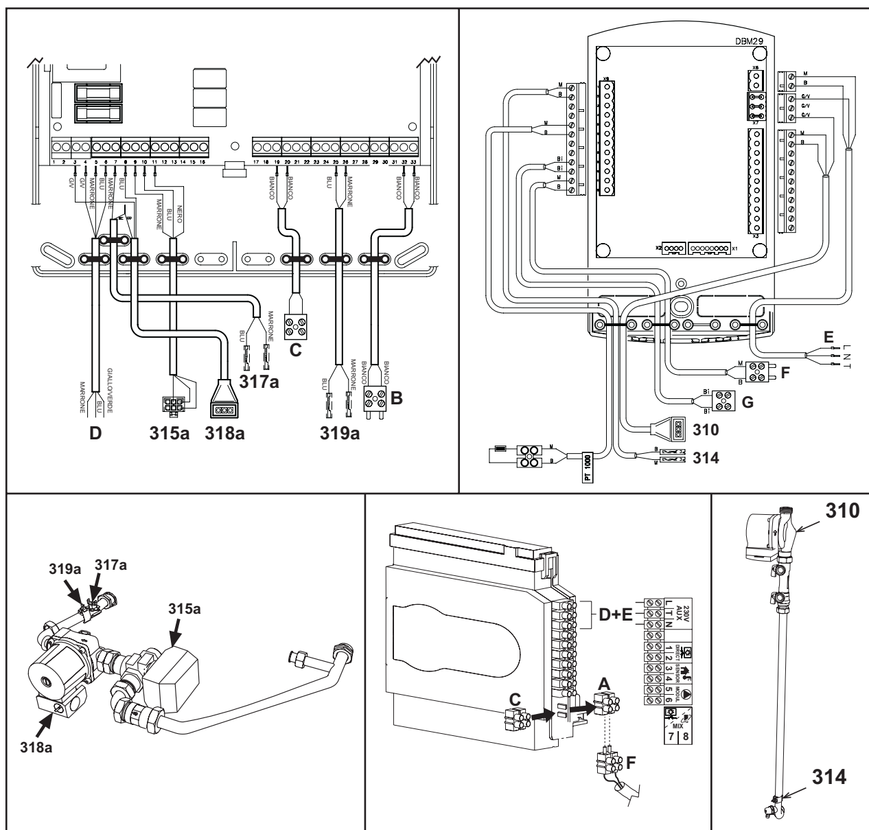
fig. 33 - Collegamenti elettrici
