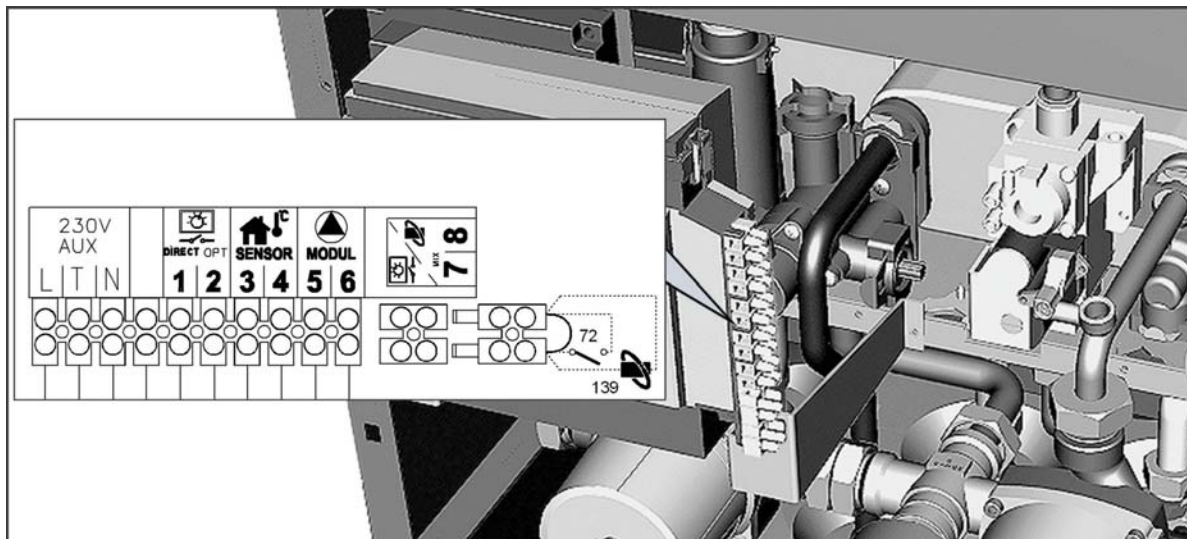
fig. 18 - Accesso alla morsettiera
