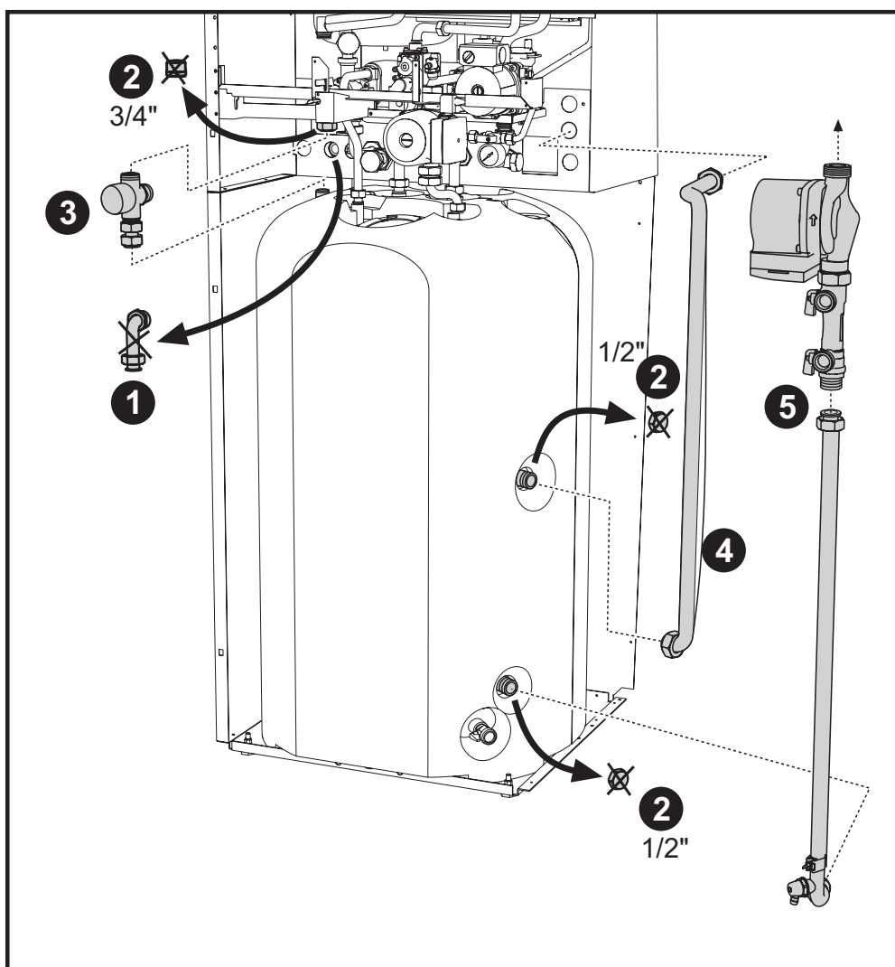
fig. 29 - Installazione Kit Solare
