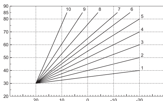
fig. 52 - Curve di compensazione
