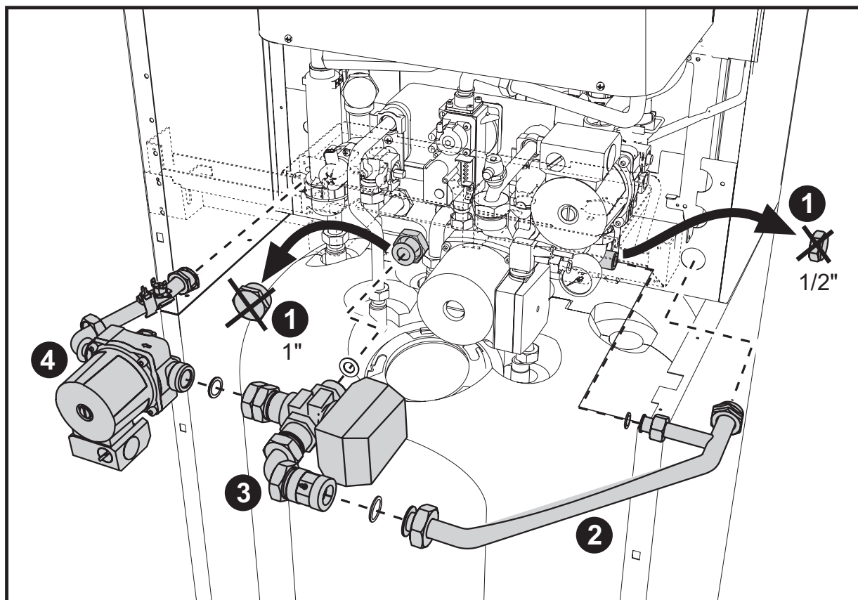
fig. 26 - Installazione Kit Bassa Temperatura
