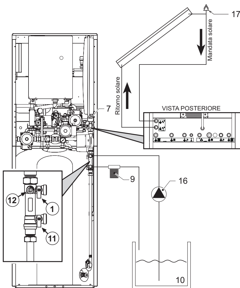
fig. 36 - Circuito solare
