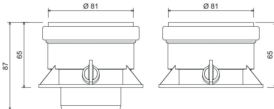
fig. 23 - Accessorio (cod. 041039X0) di partenza per condotti separati
