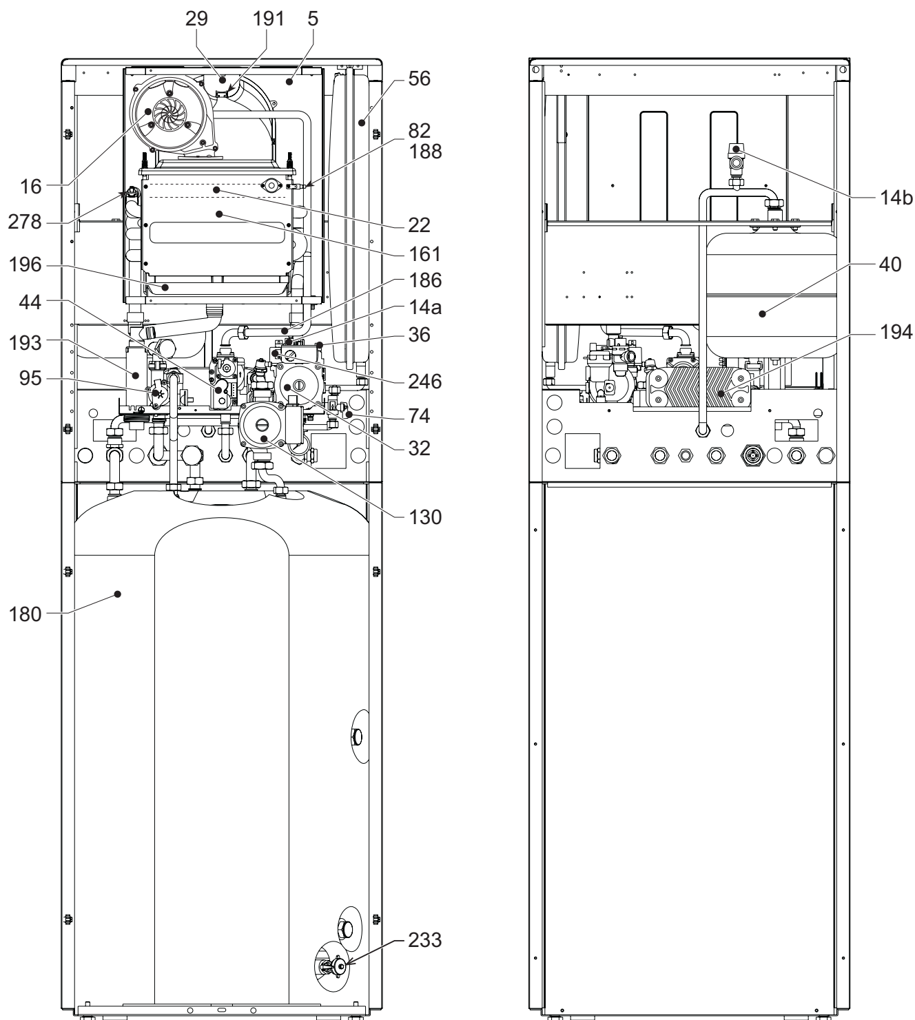
fig. 44 - Componenti principali
