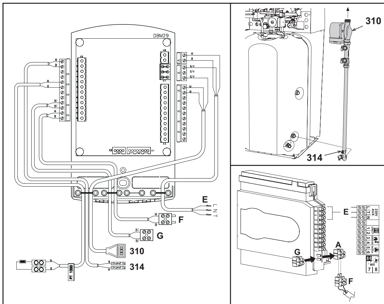
fig. 32 - Collegamenti elettrici
