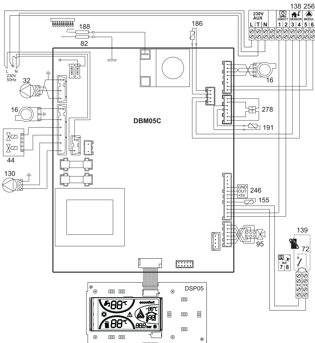
fig. 46 - Schema elettrico di serie
