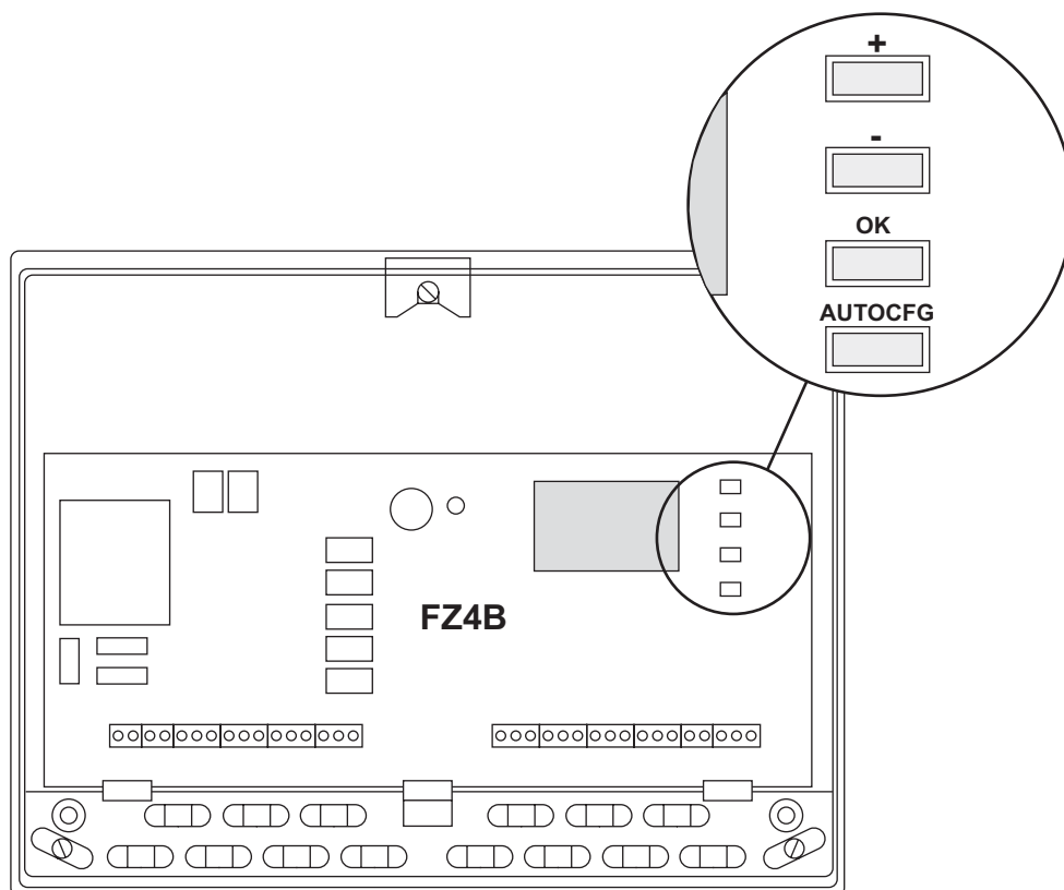
fig. 50 - Centralina FZ4B
