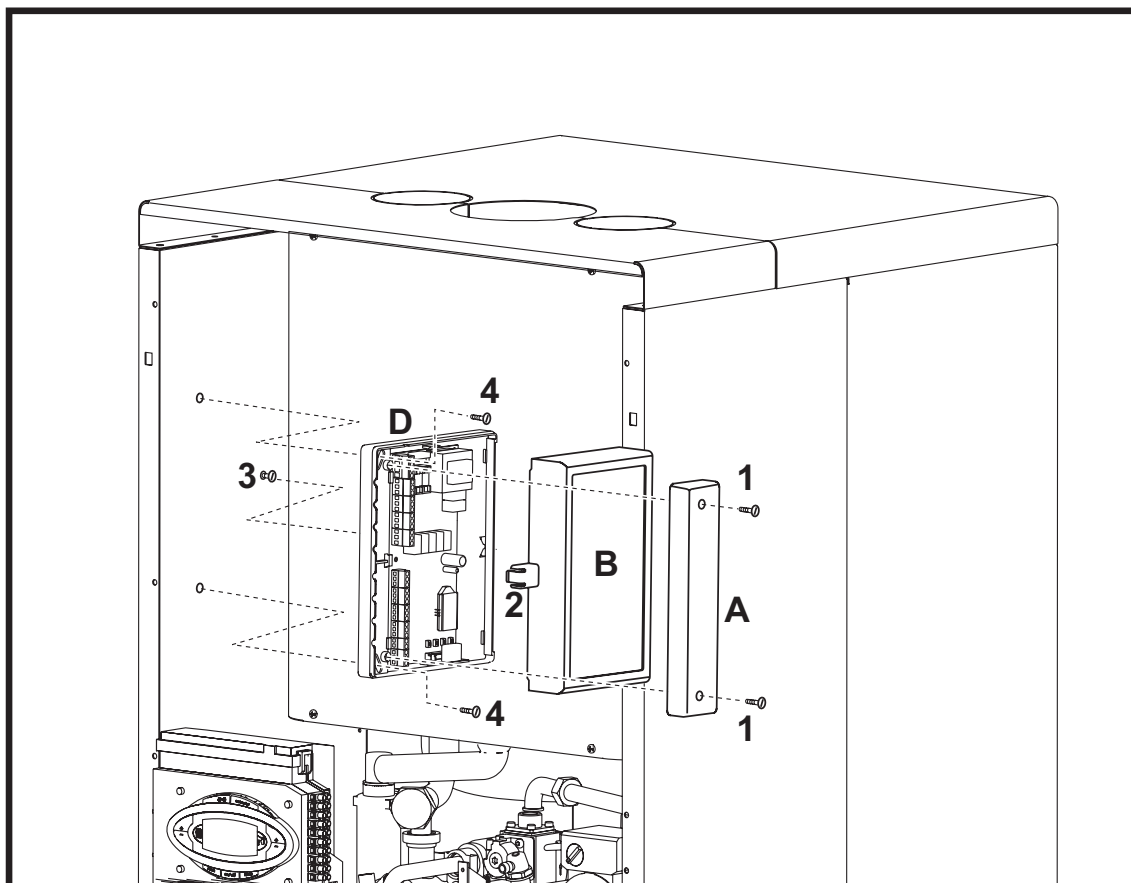
fig. 27 - Montaggio centralina
