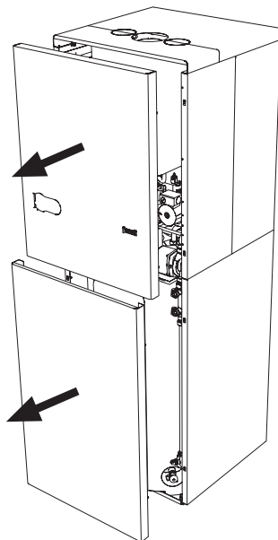
fig. 41 - Apertura mantello
