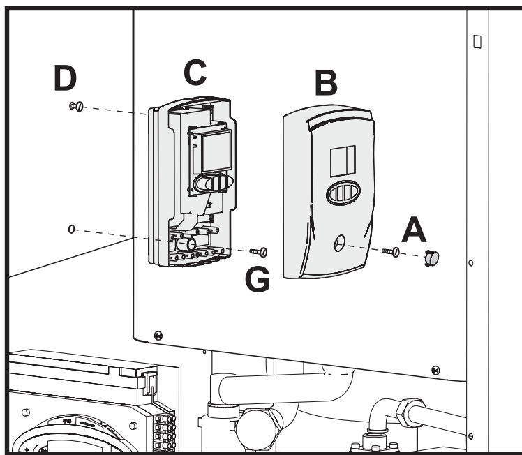
fig. 31 - Montaggio centralina
