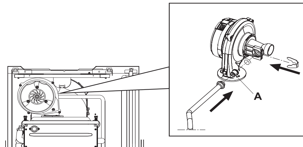
fig. 34 - Sostituzione ugello gas
