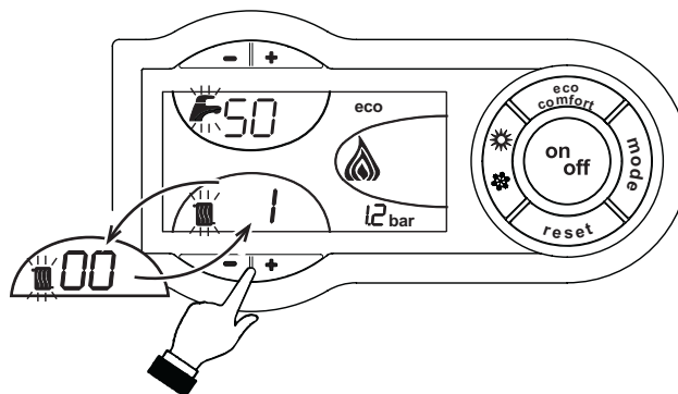
fig. 35 - Modalità TEST (potenza riscaldamento = 100%)
