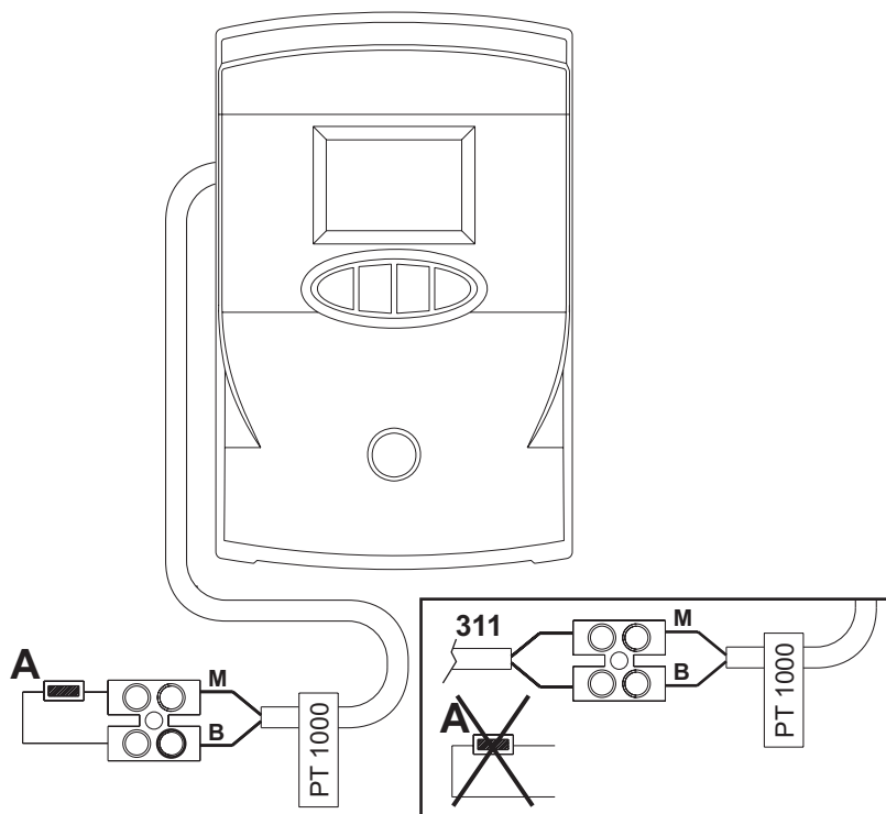
fig. 40 - Collegamento sensore collettore solare
