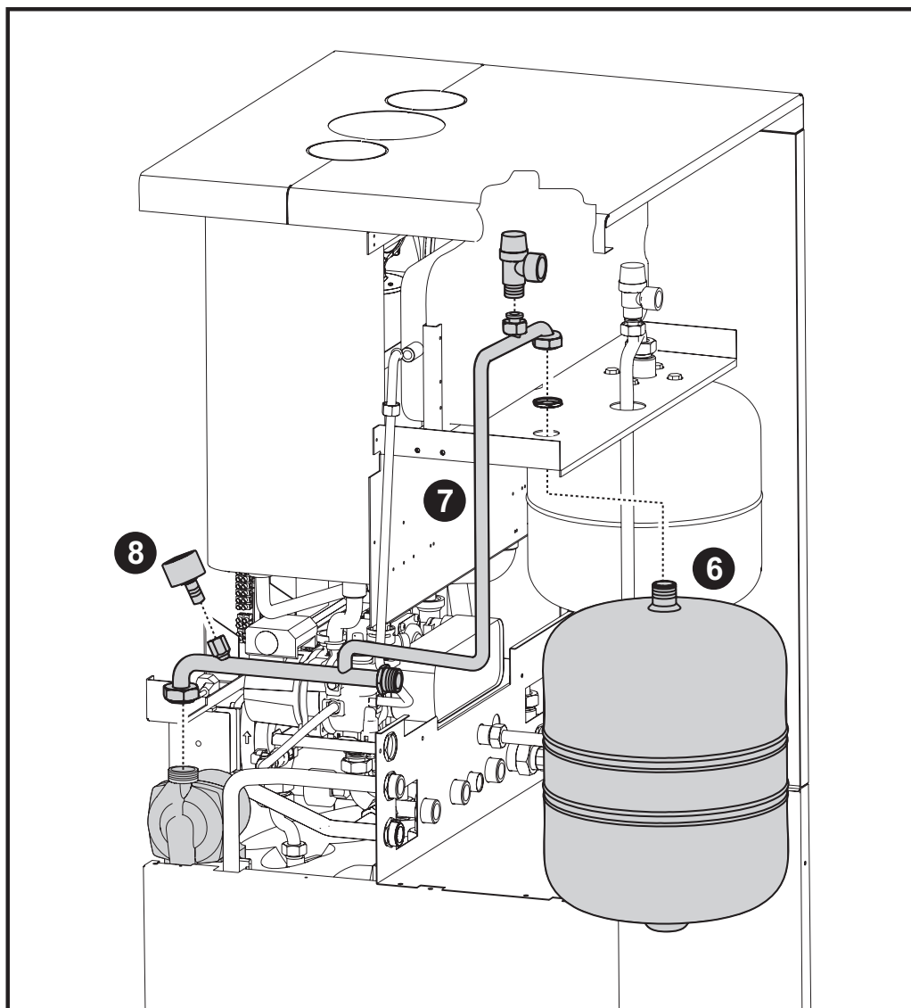
fig. 30 - Installazione Kit Solare
