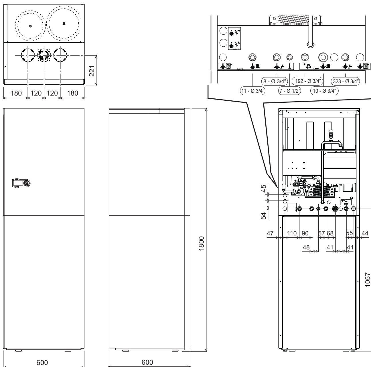
fig. 43 - Dimensioni e attacchi
