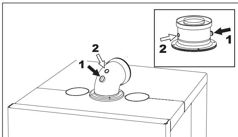
fig. 42 - Analisi della combustione
