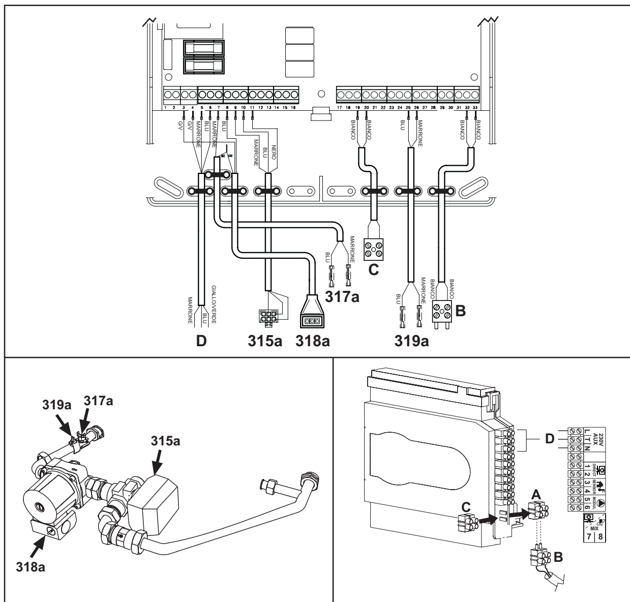
fig. 28 - Collegamenti elettrici
