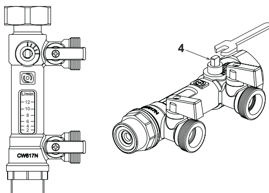
fig. 39 - Limitatore di portata
