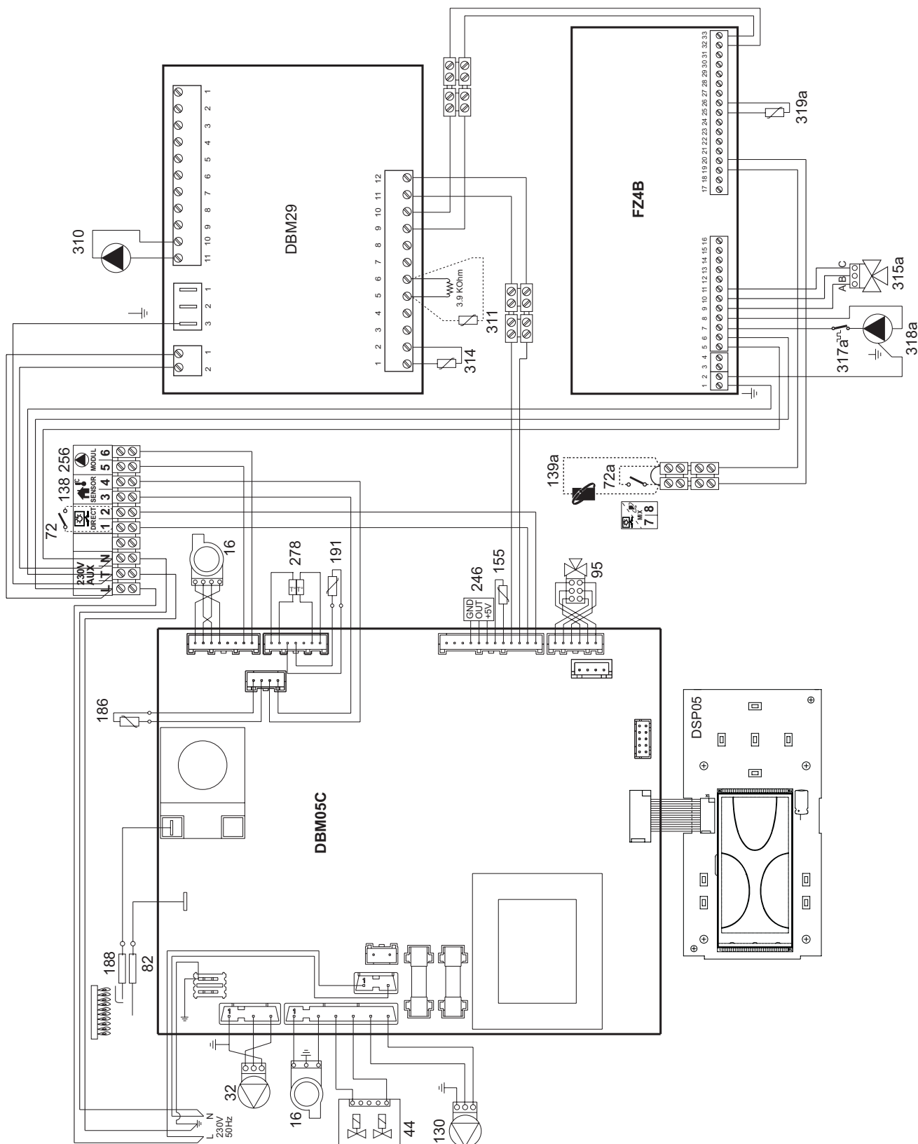
fig. 49 - Schema elettrico con solare e zona bassa temperatura
